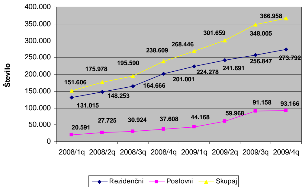
Graf št. 2: Rast IP telefonskih priključkov
