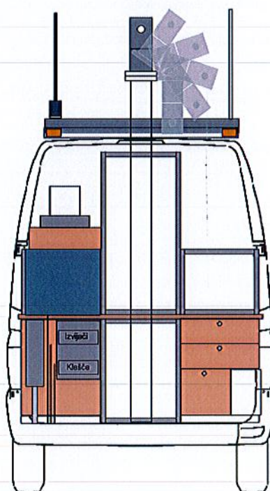
Slika 6; vozilo – pogled zadaj
