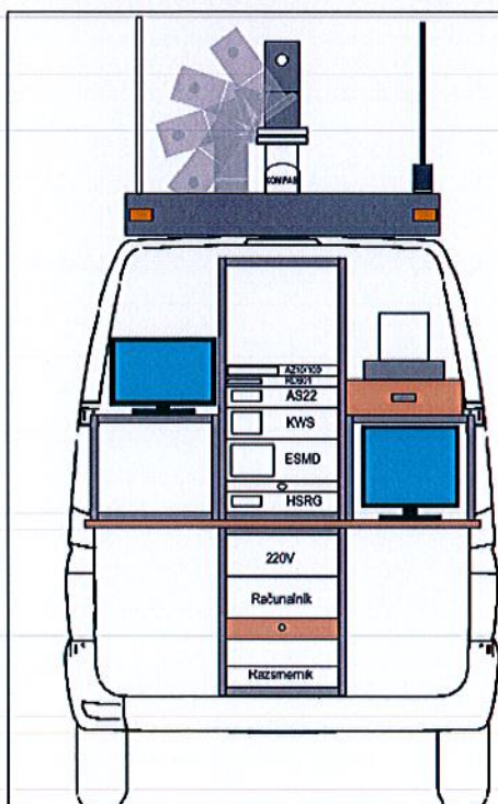
Slika 5; vozilo – pogled spredaj
